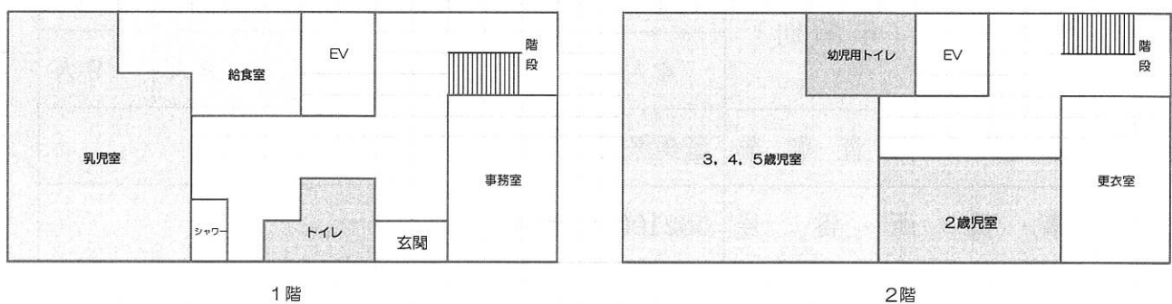
園舎平面図
